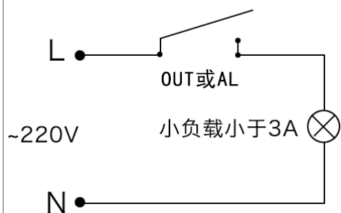
ALM 继电器接负载示意图
